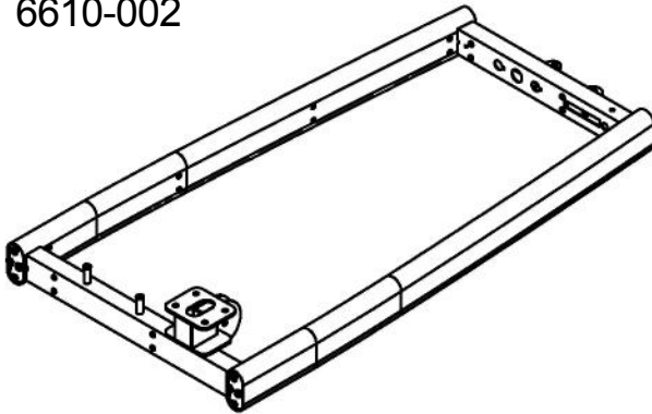
AA[1 шт] 6610-002
