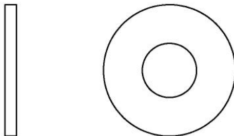
(CC1)1/2"(I.D.) Плоская шайба Ø34, 4 шт.
