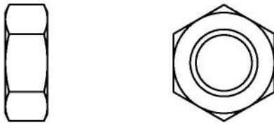
(BB1) Гайка 1/2"-13UNC, 1 шт.
