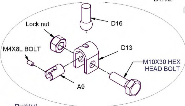
B詳圖
